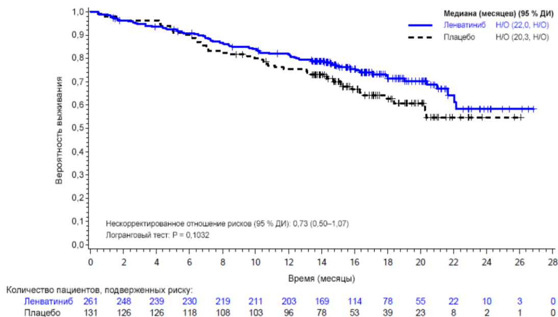
Рисунок 2. График Каплана-Мейера для общей выживаемости (ДРЩЖ)
