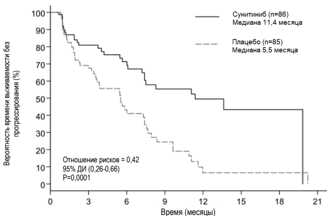
Рисунок 1. Кривая Каплана-Мейера для ВБП в исследовании НЭОПЖ 3 фазы
